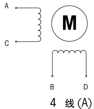
接线图(Wiring Diagram):
